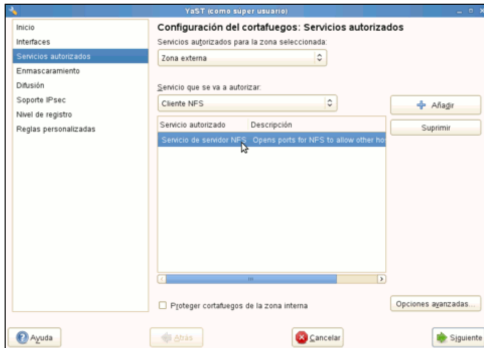
Módulo de cortafuegos de YaST, en modo gráfico, habilitando el Servicio de Servidor NFS .
