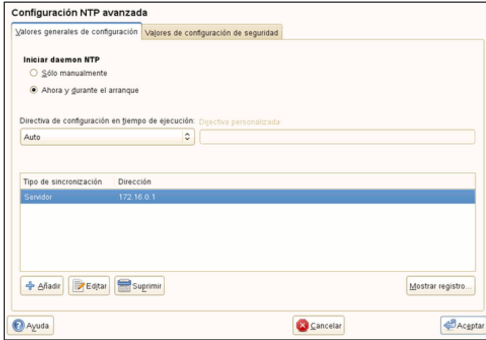
Módulo de Cliente NTP de YaST, en modo gráfico.
