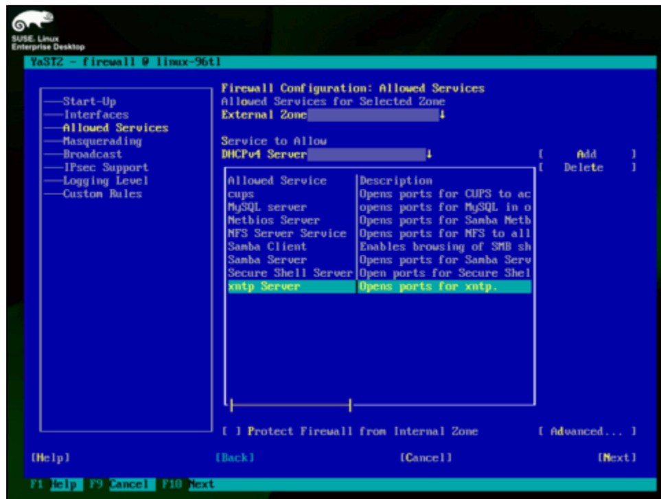
Módulo de cortafuegos de YaST, en modo texto, habilitando nntp Server.
