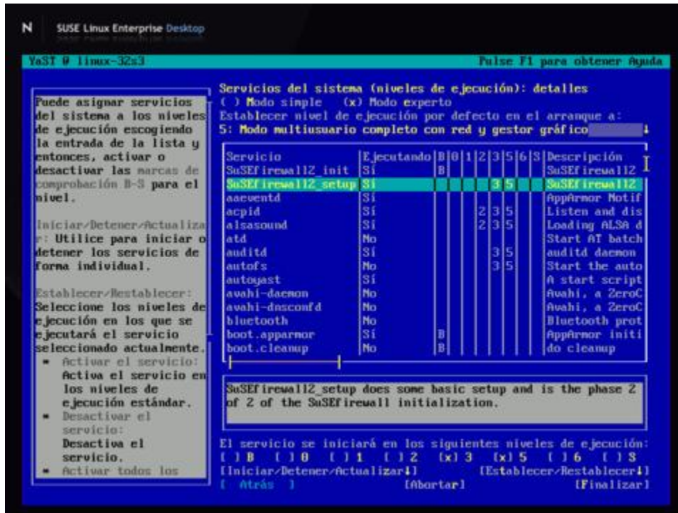
Módulo runlevel de YaST, en modo experto.
