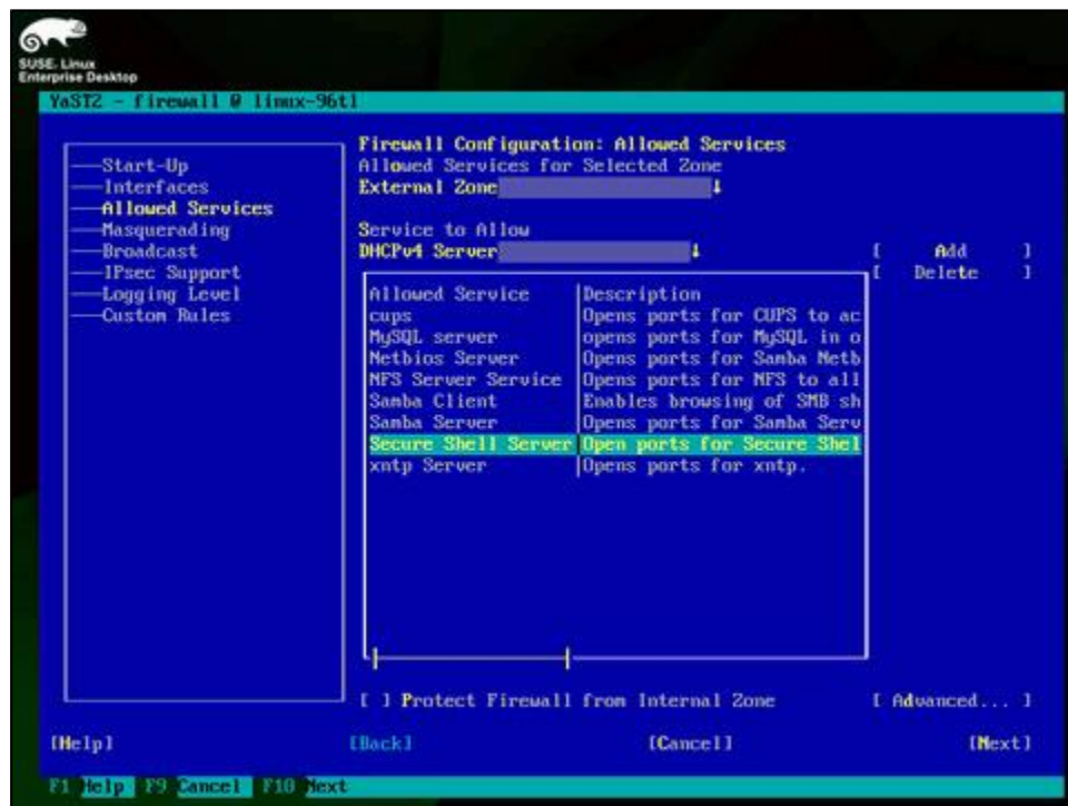
Módulo de cortafuegos de YaST, habilitando Secure Shell Server.
