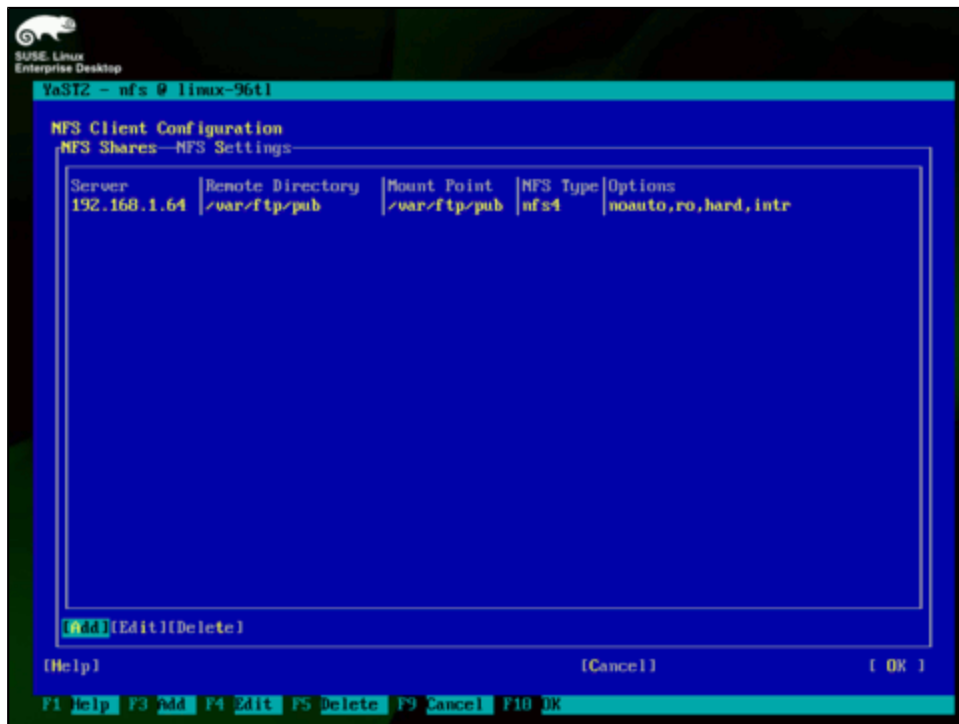
Módulo de nfs de YaST, en modo texto.
