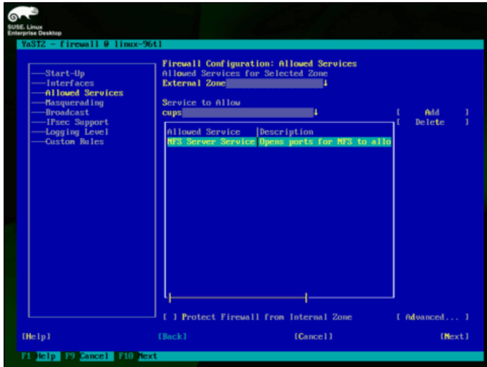
Módulo de cortafuegos de YaST, en modo texto, habilitando NFS Server Service .
