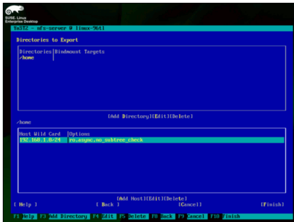
Módulo nfs-server de YaST.
