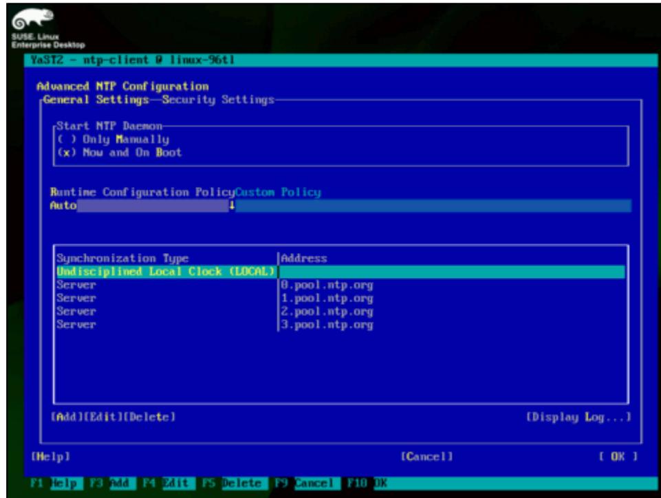
Módulo de Cliente NTP de YaST, en modo texto, configurando como servidor NTP.
