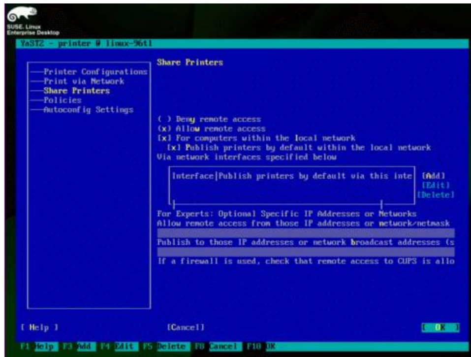
Módulo de Impresoras de YaST en modo terminal.
