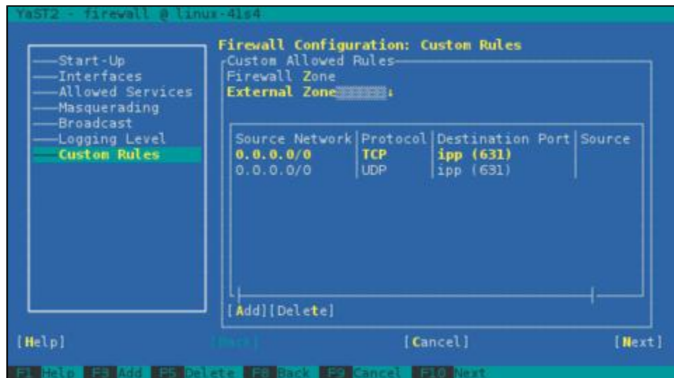
Módulo de cortafuegos de YaST, en modo texto, habilitando el puerto 631 por TCP y UDP.
