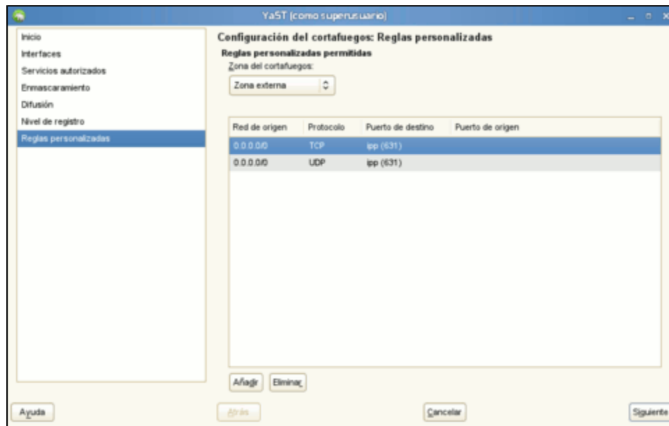
Módulo de cortafuegos de YaST, en modo gráfico, habilitando el puerto 631 por TCP y UDP.
