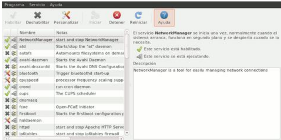
Herramienta system-config-services.
