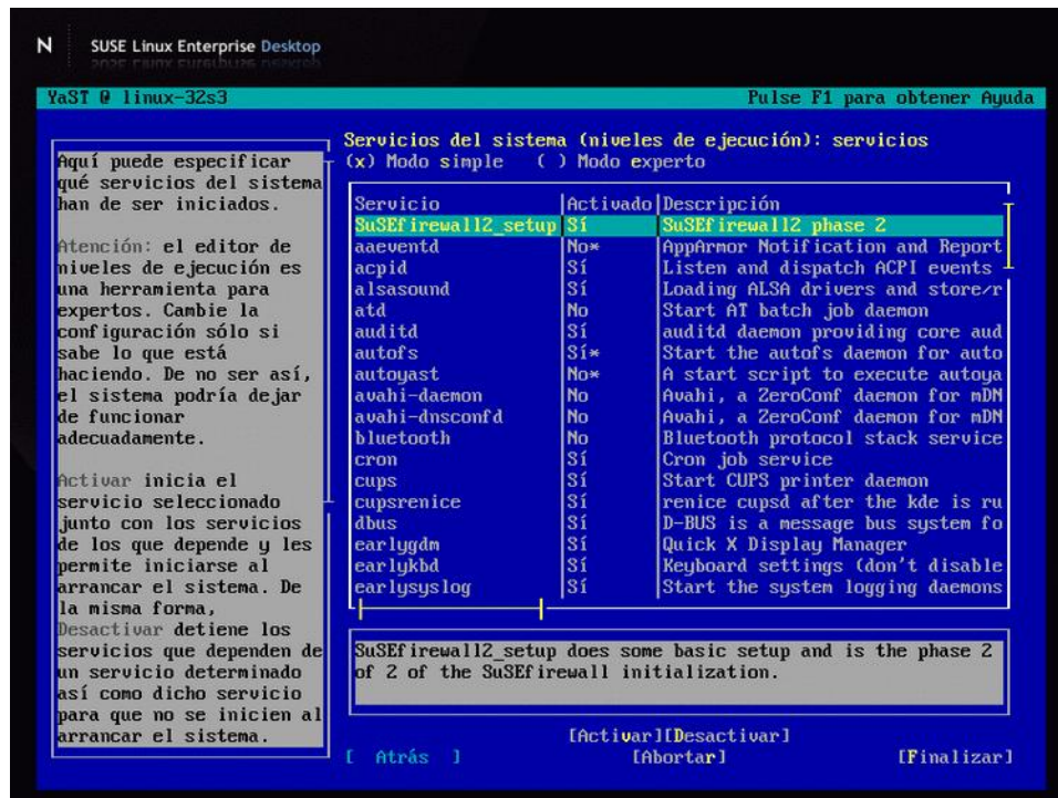
Módulo runlevel de YaST, en modo simple.
