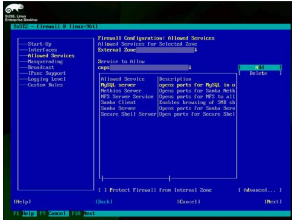
Módulo de cortafuegos de YaST, en modo texto, habilitando MySQL Server .
