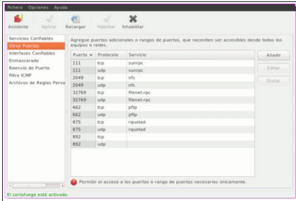
System-config-firewall habilitando puertos para NFS.
